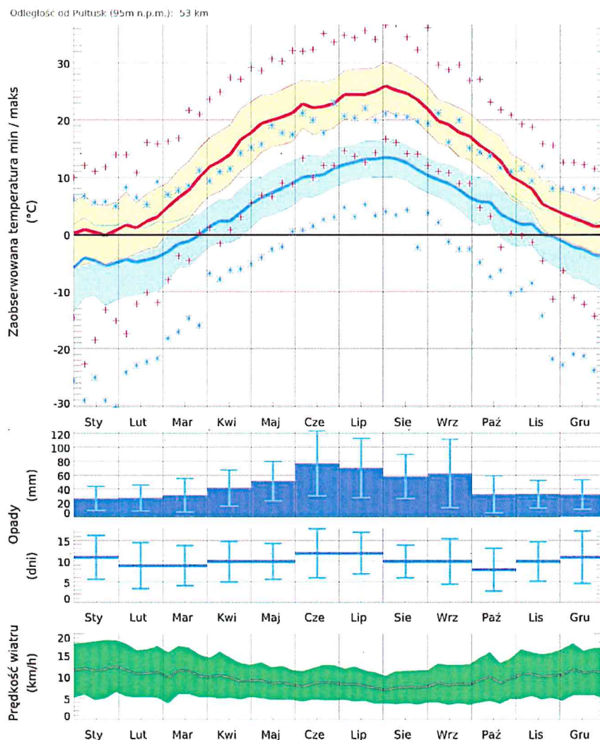
Rycina 3. Meteogram dla Powiatu Pułtuskiego
